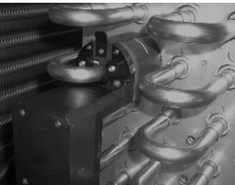
Optimale Lösung zum Verschweißen von vormontierten Bögen. Geringster Platzbedarf durch kompakte Bauform.
